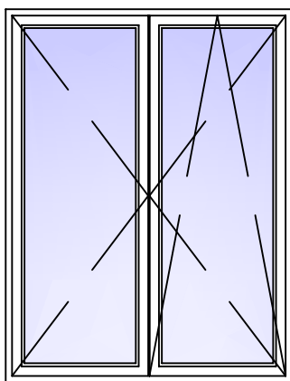
Középen felnyíló bukó-nyíló erkélyajtó
